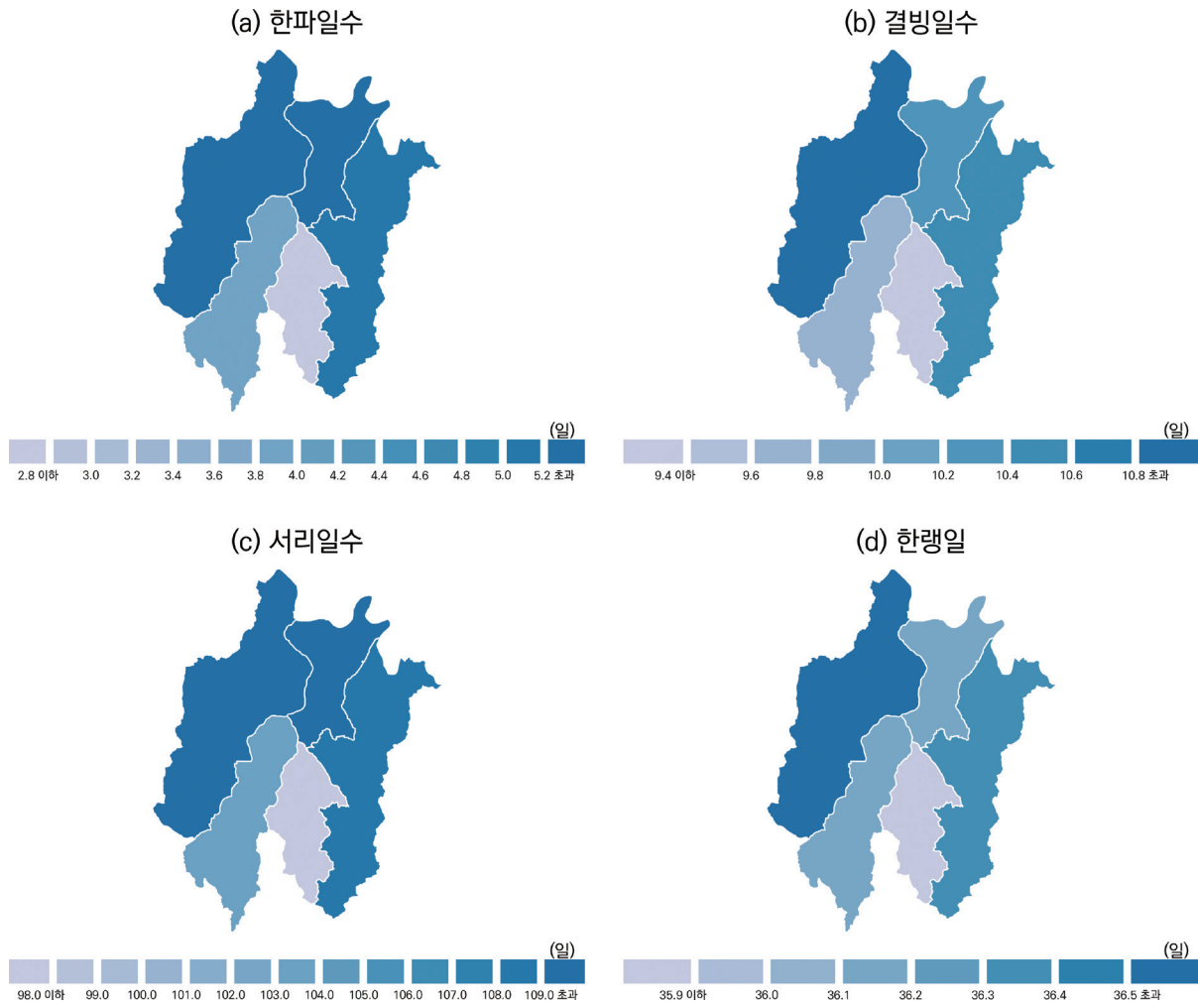
그림 3-3. 현재(2000-2019년) 대전광역시 저온 관련 극한기후지수 분포
