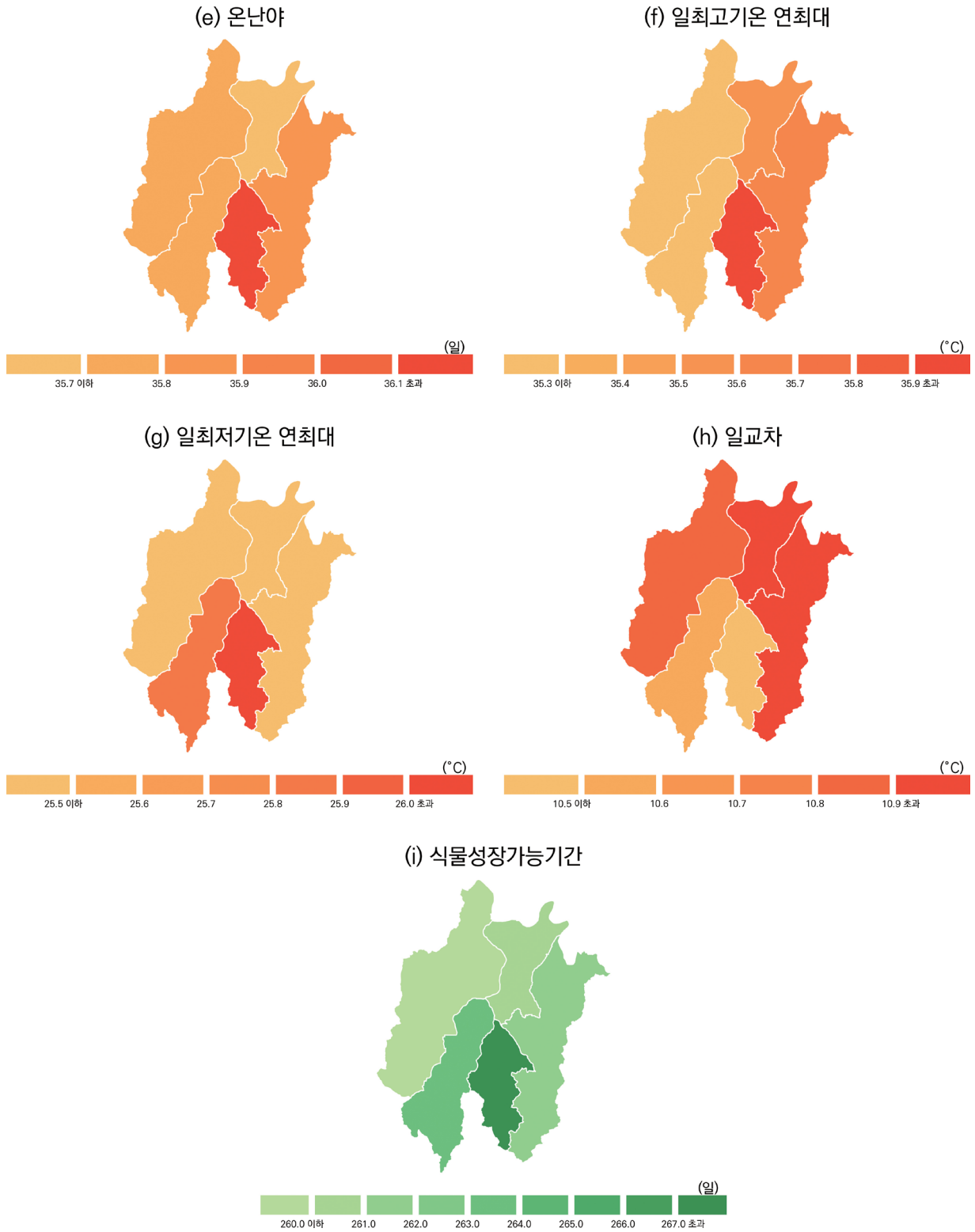
그림 3-2. 현재(2000-2019년) 대전광역시 고온 관련 극한기후지수 분포(계속)
