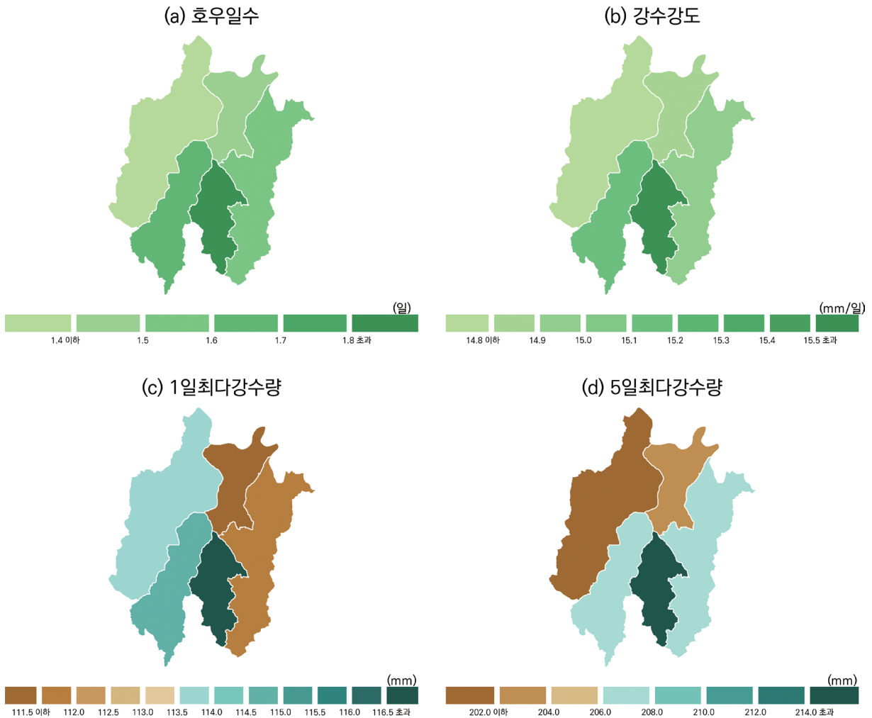
그림 3-4. 현재(2000-2019년) 대전광역시 강수 관련 극한기후지수 분포
