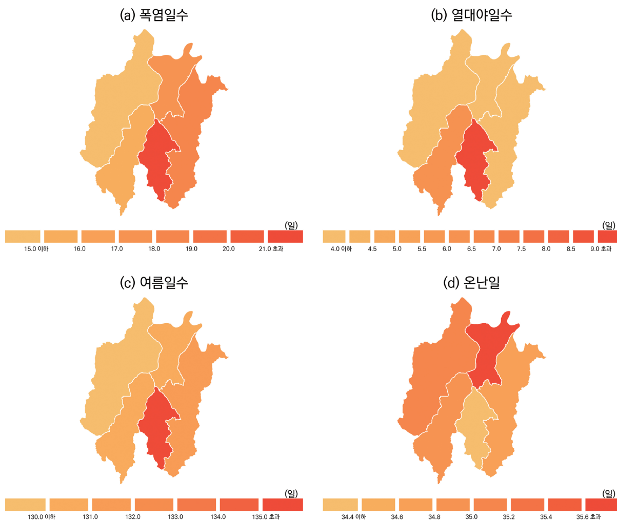
그림 3-2. 현재(2000-2019년) 대전광역시 고온 관련 극한기후지수 분포
