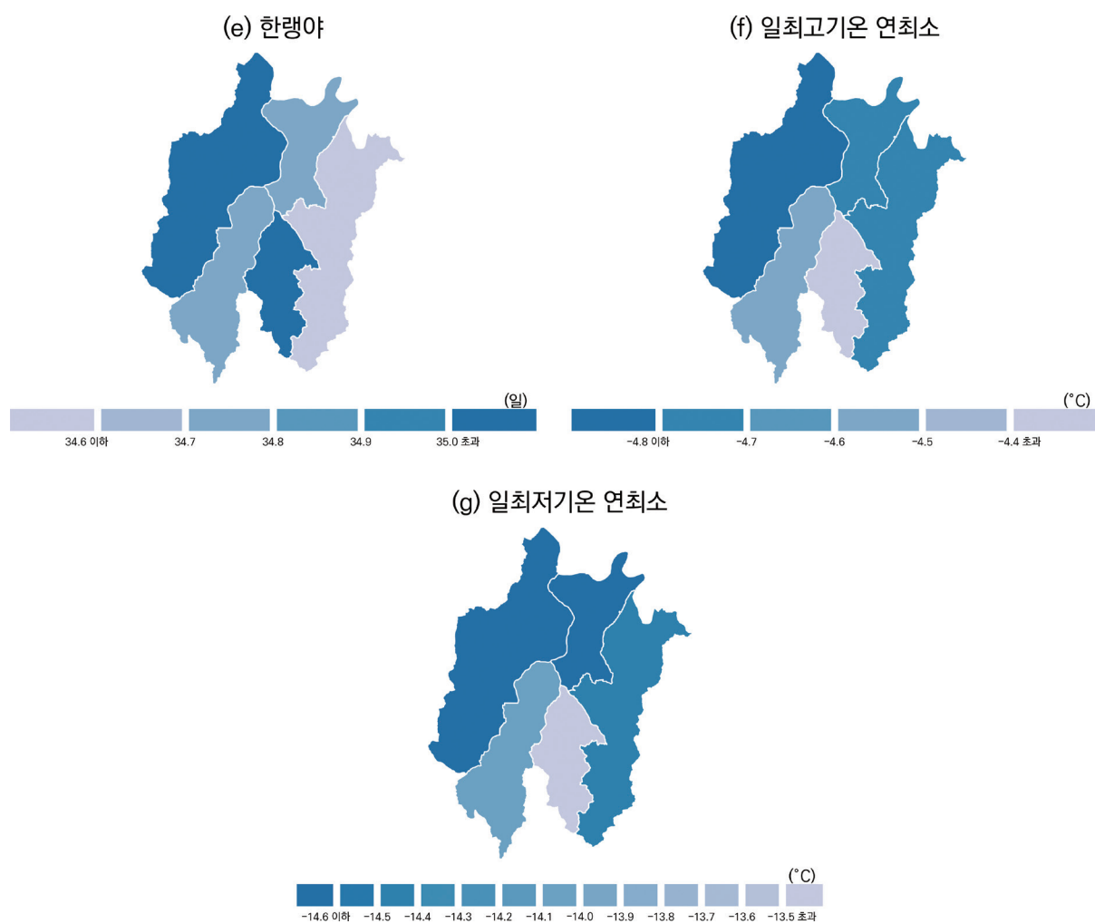
그림 3-3. 현재(2000-2019년) 대전광역시 저온 관련 극한기후지수 분포(계속)
