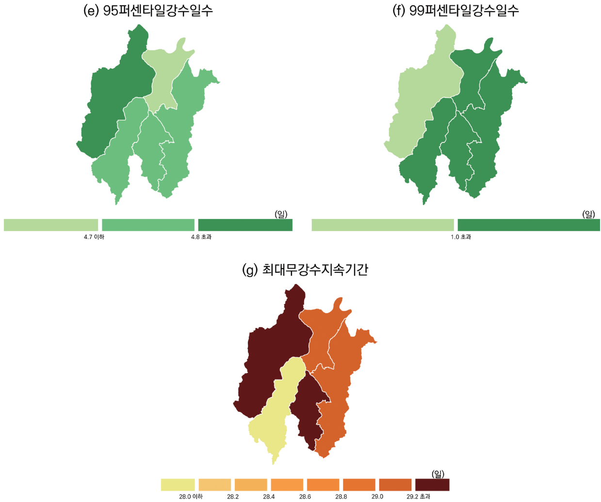
그림 3-4. 현재(2000-2019년) 대전광역시 강수 관련 극한기후지수 분포(계속)
